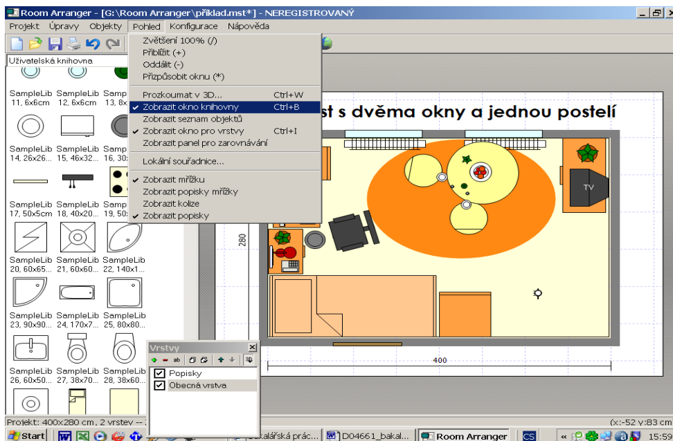
Uživatelská knihovna.
