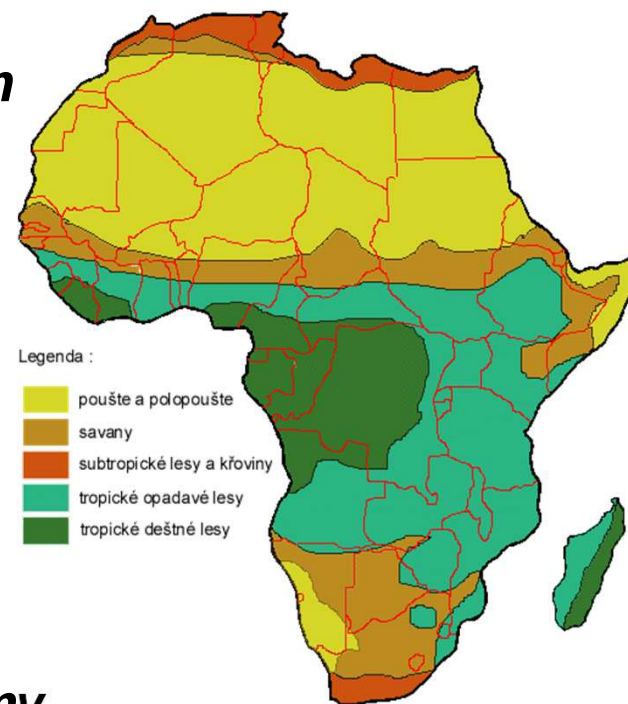
obr.2 Schematická mapa přírodních krajín Afriky
